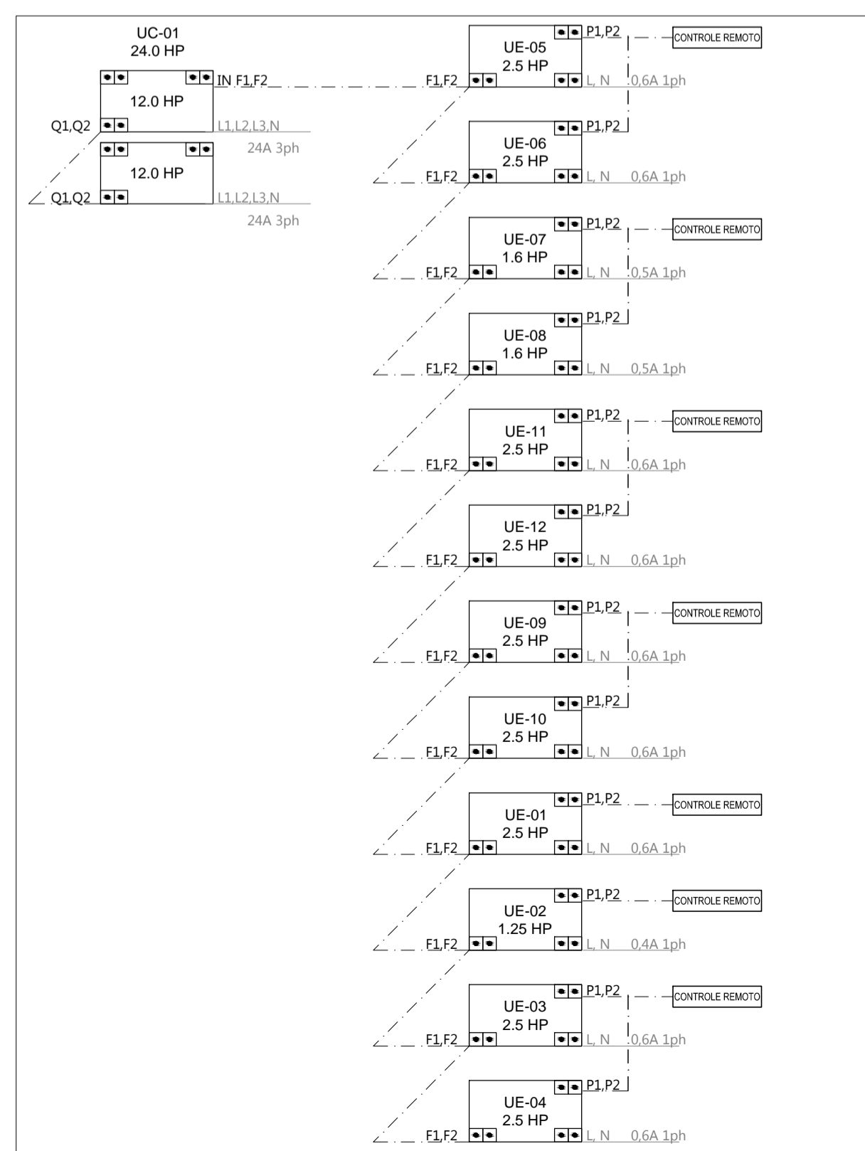
07 DIAGRAMA ELÉTRICO E DE COMANDO SEM ESCALA
